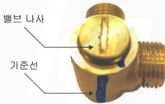
유량조절밸브(지수밸브)
